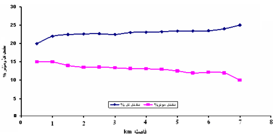
شکل ۶- دیاگرام تغییرات تخلخل کل و موثر رسوبات آبرفت رودخانه در آبراه اصلی
