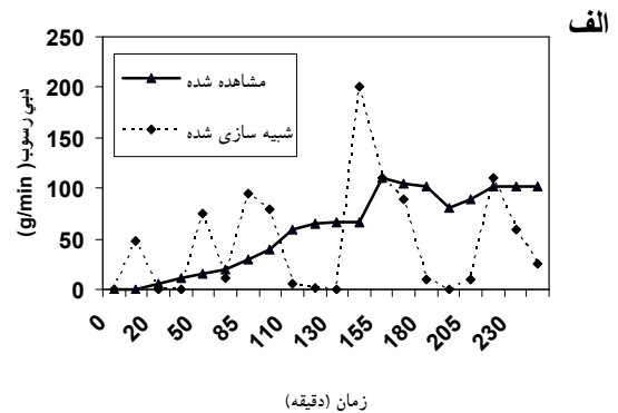
شکل ۵. منحنی واسنجی رسوب- زمان برای رخداد ۲۶ فروردین ۱۳۸۲ قبل (الف) و بعد (ب) از واسنجی به وسیله مدل EUROSEM در حوضه سولیمانجان
