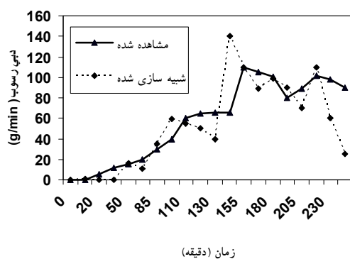
شکل ۵. منحنی واسنجی رسوب- زمان برای رخداد ۲۶ فروردین ۱۳۸۲ قبل (الف) و بعد (ب) از واسنجی به وسیله مدل EUROSEM در حوضه سولیمانجان
