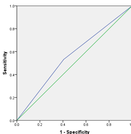
شکل ۱. منحنی ROC برای آزمایش سرولوژی
