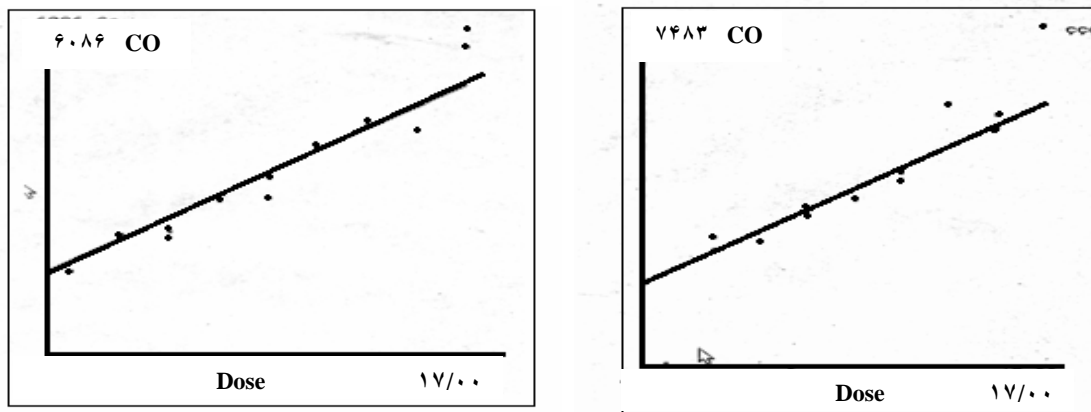
شکل ۱. کالبراسیون گروهی کانال A و B. در این نمودار، محور افقی مقادیر دوز داده شده به هر گروه است و محور عمودی، میانگین شمارش تصحیح شده ضرب در فاکتور کالبراسیون فردی مربوطه به هر دوزیمتر است که برای هر ۳ دوزیمتر مربوط به یک گروه محاسبه شد. فاکتور کالبراسیون گروهی با استفاده از شیب و مقدار دوز زمینه با استفاده از قطع محور دوز توسط خط به دست آمد.
