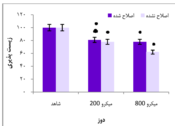
شکل ۴. مقایسه‌ی نانو میله‌های اکسید آهن اصلاح شده و نشده با یکدیگر و کنترل در ۷۲ ساعت •: مقایسه‌ی هر دوز با کنترل ( P < 0/05 ), ♣: مقایسه‌ی دوز ۲۰۰ μg/ml با ۸۰۰ μg/ml ( P < 0/05 ), ستون‌ها نمایانگر میانگین ± دامنه‌ی تغییرات می‌باشد.
