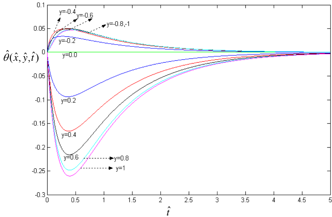
شکل ۱- نمودار تغییرات دمای بدون بعد با زمان در بارگذاری ترکیبی در مسئله اول B.C1-I.C1 ، x=0.5, L=1
