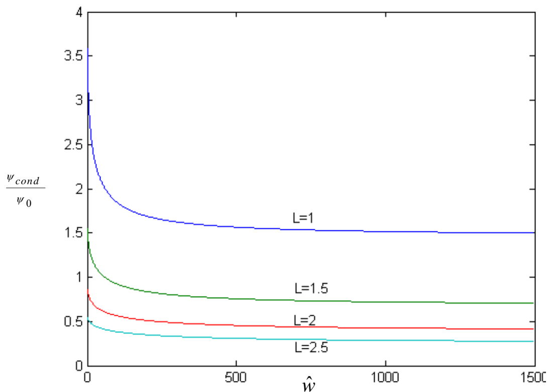
شکل ۲۰- نمودار تغییرات نسبت تولید آنتروپی ناشی از گرادیان دما به کل کار انجام شده با پارامتر \hat{w} و L در بارگذاری ترکیبی در ترموالاستیسیتیه در مسأله اول با شرایط مرزی ۱ و اولیه ۴ (نیمه بالایی)
