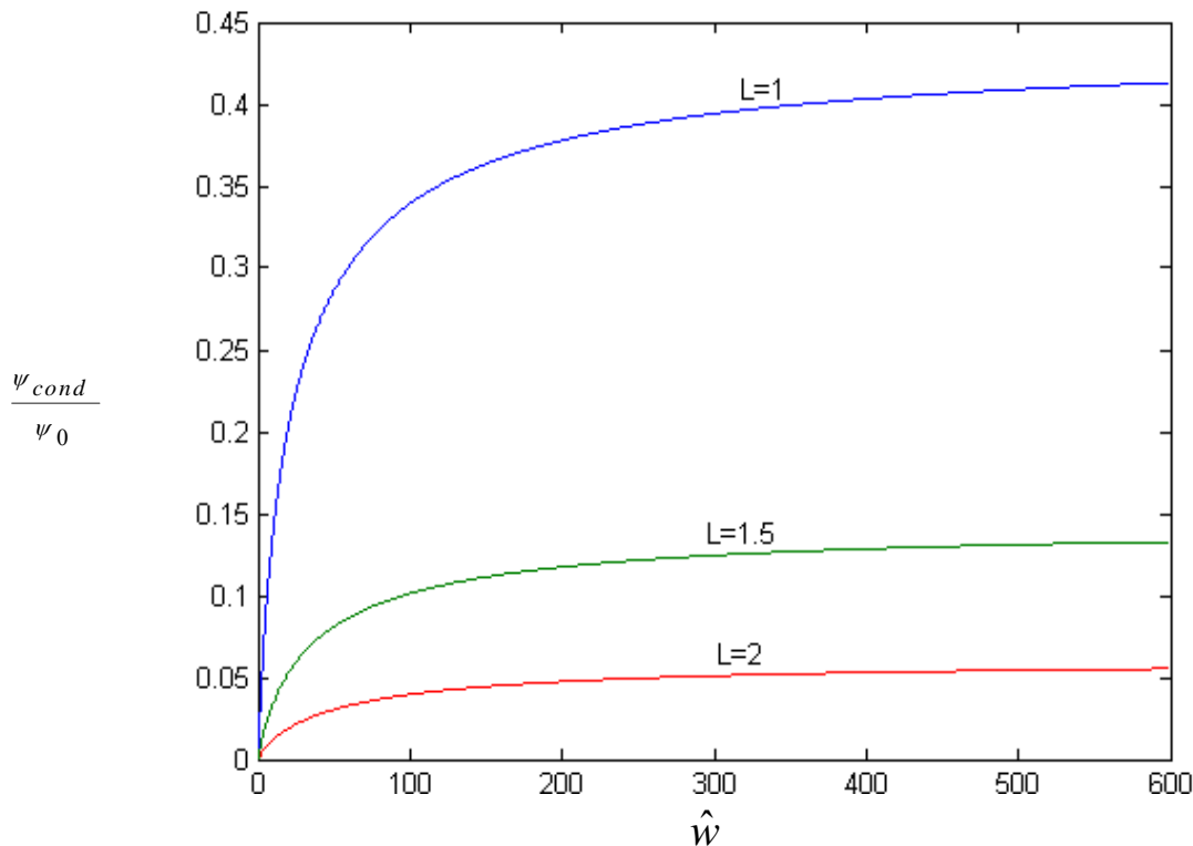
شکل ۲۳- نمودار تغییرات نسبت تولید آنتروپی ناشی از گرادیان دما به کل کار انجام شده با پارامتر \hat{w} و L در بارگذاری ترکیبی در ترموالاستیسیتیه در مسأله اول با شرایط مرزی ۲ و اولیه ۱ (نیمه پایینی)
