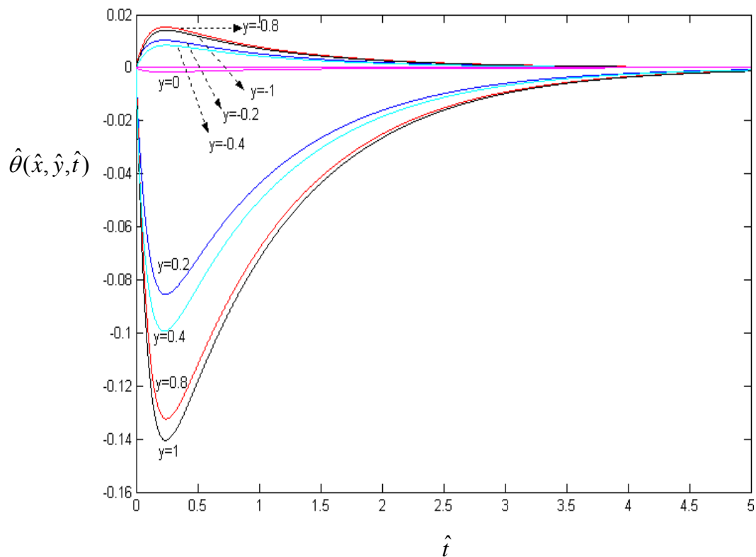
شکل ۵- نمودار تغییرات دمای بدون بعد با زمان در بارگذاری ترکیبی در مسأله اول B.C2-I.C1 ، x=0.5, L=1
