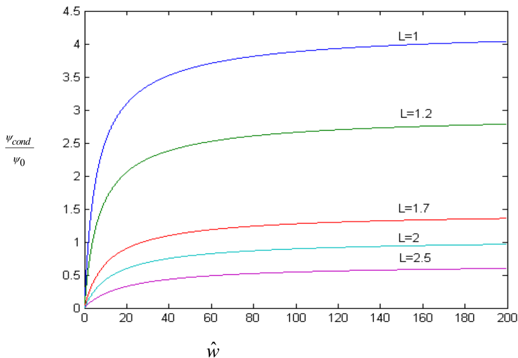
شکل ۱۳- نمودار تغییرات نسبت تولید آنتروپی ناشی از گرادیان دما به کل کار انجام شده با پارامتر \hat{w} و L در بارگذاری ترکیبی در ترموالاستیسیته در مسأله اول با شرایط مرزی ۱ و اولیه ۱ (نیمه بالایی)
