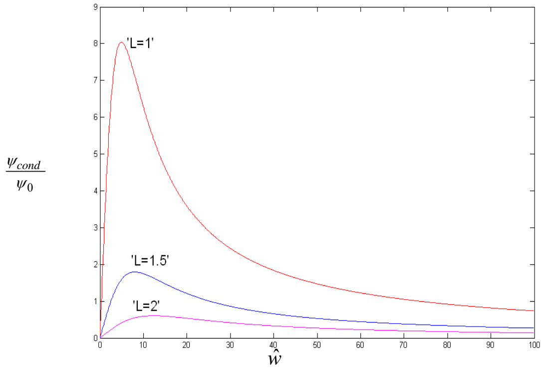
شکل ۳۱ - نمودار تغییرات نسبت تولید آنتروپی ناشی از گرادیان دما به کل کار انجام شده با پارامتر \hat{\omega} و L در بارگذاری ترکیبی متناوب در ترموالاستیسیته در مسأله دوم با شرایط مرزی ۲ و اولیه ۱
