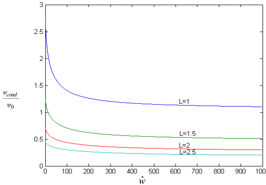
شکل ۱۹- نمودار تغییرات نسبت تولید آنتروپی ناشی از گرادیان دما به کل کار انجام شده با پارامتر \hat{w} و L در بارگذاری ترکیبی در ترموالاستیسیتیه در مسأله اول با شرایط مرزی ۱ و اولیه ۳ (نیمه پایینی)
