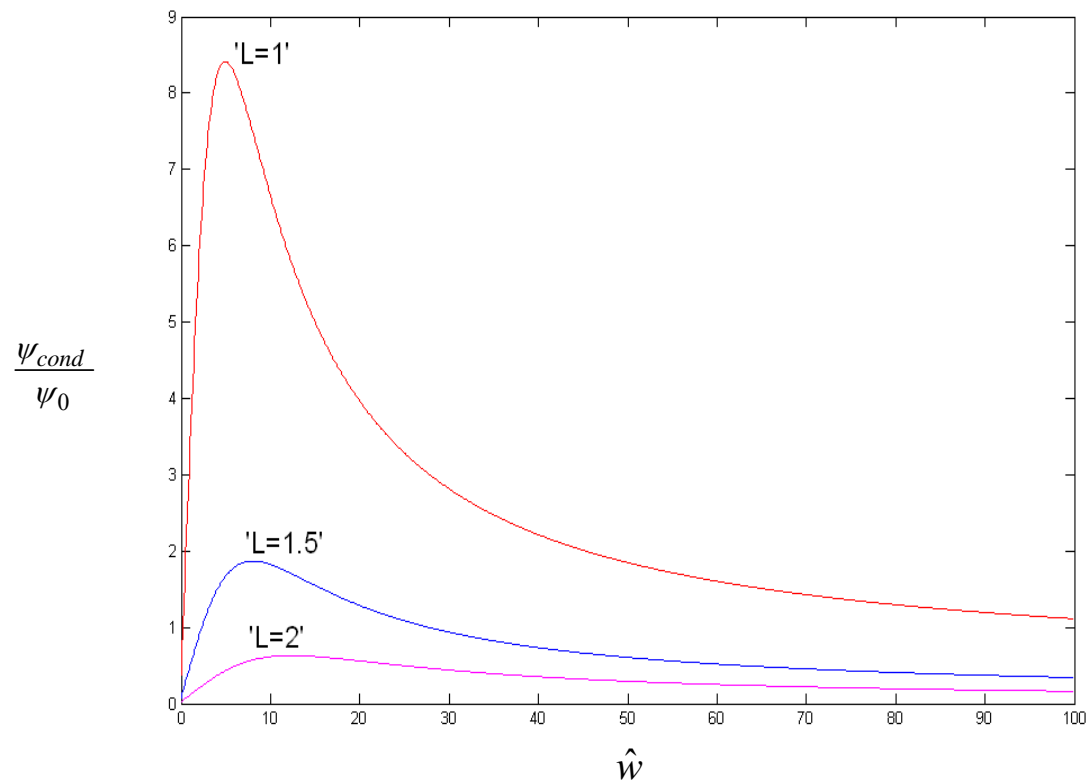
شکل ۳۴- نمودار تغییرات نسبت تولید آنتروپی ناشی از گرادیان دما به کل کار انجام شده با پارامتر \hat{w} و L در بارگذاری ترکیبی متناوب در ترموالاستیسیتیه در مسأله دوم با شرایط مرزی ۲ و اولیه ۴
