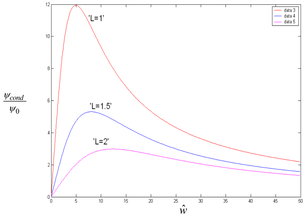
شکل ۲۷- نمودار تغییرات نسبت تولید آنتروپی ناشی از گرادیان دما به کل کار انجام شده با پارامتر \hat{w} و L در بارگذاری ترکیبی متناوب در ترموالاستیسیتیه در مسأله دوم با شرایط مرزی ۱ و اولیه ۱
