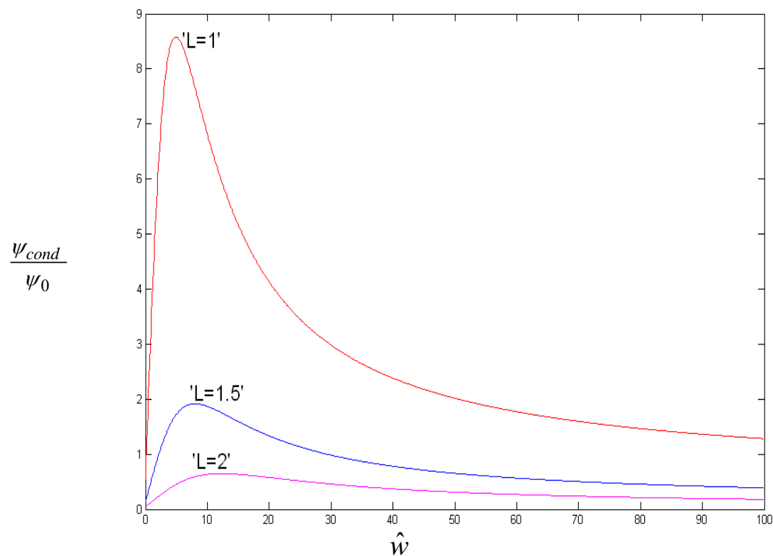
شکل ۳۳- نمودار تغییرات نسبت تولید آنتروپی ناشی از گرادیان دما به کل کار انجام شده با پارامتر \hat{w} و L در بارگذاری ترکیبی متناوب در ترموالاستیسیتیه در مسأله دوم با شرایط مرزی ۲ و اولیه ۳
