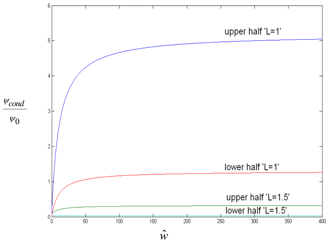
شکل ۲۴- نمودار تغییرات نسبت تولید آنتروپی ناشی از گرادیان دما به کل کار انجام شده با پارامتر \hat{w} و L در بارگذاری ترکیبی در ترموالاستیسیتیه در مسأله اول با شرایط مرزی ۲ و اولیه ۲
