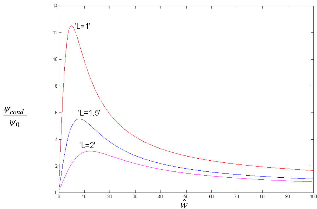
شکل ۳۰ - نمودار تغییرات نسبت تولید آنتروپی ناشی از گرادیان دما به کل کار انجام شده با پارامتر \hat{w} و L در بارگذاری ترکیبی متناوب در ترموالاستیسیته در مسأله دوم با شرایط مرزی ۱ و اولیه ۴
