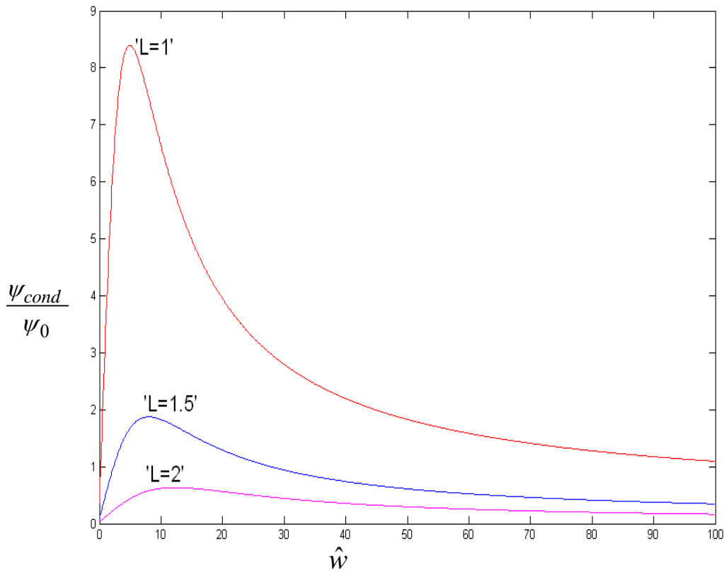
شکل ۳۲ - نمودار تغییرات نسبت تولید آنتروپی ناشی از گرادیان دما به کل کار انجام شده با پارامتر \hat{\omega} و L در بارگذاری ترکیبی متناوب در ترموالاستیسیته در مسأله دوم با شرایط مرزی ۲ و اولیه ۲
