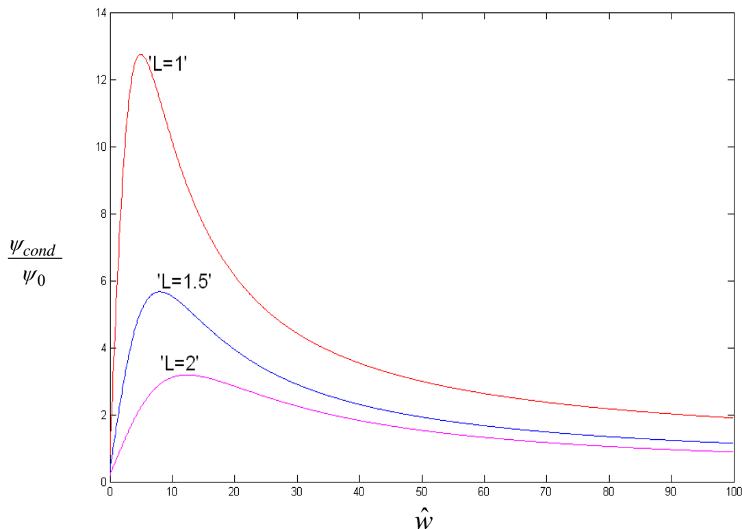
شکل ۲۹ - نمودار تغییرات نسبت تولید آنتروپی ناشی از گرادیان دما به کل کار انجام شده با پارامتر \hat{w} و L در بارگذاری ترکیبی متناوب در ترموالاستیسیته در مسأله دوم با شرایط مرزی ۱ و اولیه ۳
