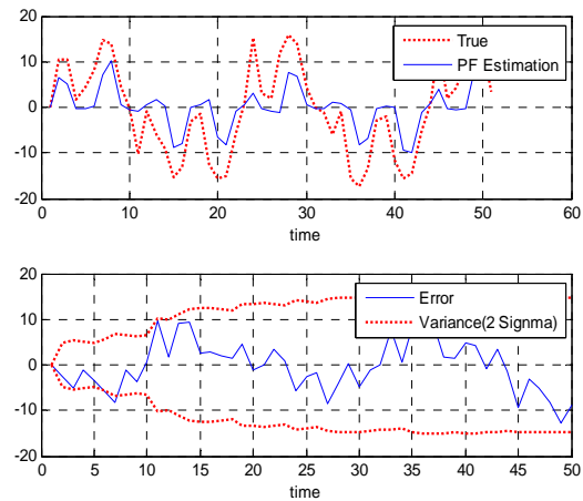
شکل (۱۲): فیلتر ذره‌ای (N=100).
