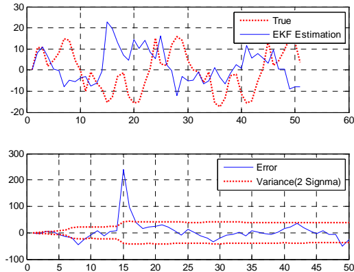
شکل (۱۱): فیلتر کالمن توسعه یافته (EKF).
