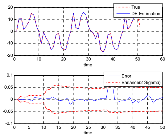
شکل (۶): فیلتر مبتنی بر تکامل تفضلی (N=100).
