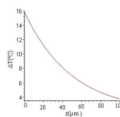
نمودار ۳ ب: تغییرات دما بر حسب عمق برای انرژی ۲/۴ ژول
