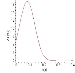
نمودار ۳ الف: تغییرات دما بر حسب زمان برای انرژی ۲/۴ ژول
