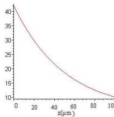
نمودار ۴ ب: تغییرات دما بر حسب عمق برای انرژی ۸ ژول
