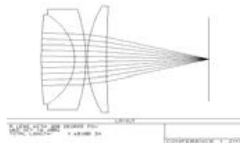
شکل ۳: سیستم اپتیکی موازی ساز به همراه جدول آن که به صورت شبه متقارن برای حذف ابیراهی های مخالف طراحی شده است.
