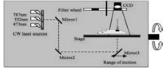
شکل ۲: تصویر شماتیکی از سیستم تصویربرداری توموگرافی فلورسنت مولکولی
