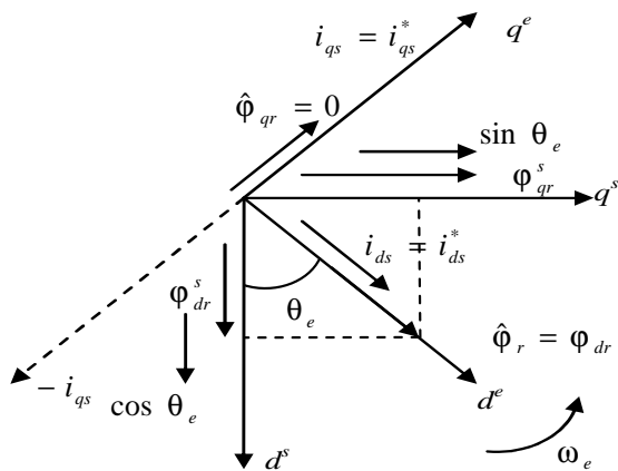
شکل (۲): دیگرام برداری مؤلفه‌های d_s - q_s و d_e - q_e [1].
