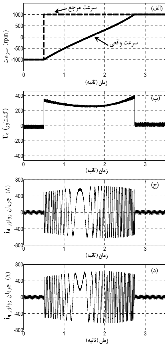
شکل (۶): نتایج شبیه سازی برای سرعت 1000 \text{ rpm} \pm بدون جبران شار روتور، الف: پروفایل سرعت روتور، ب: پروفایل گشتاور تولیدی، ج: جریان روتور بر روی محور d و د: جریان روتور بر روی محور q
