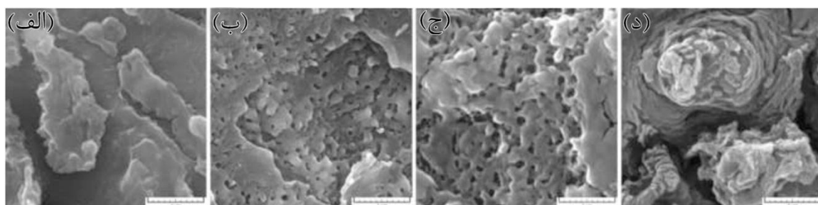
شکل ۱. تصاویر میکروسکوپی الکترونی روبشی لایه‌های رشد داده شده تحت ولتاژهای الف: ۵۰ ولت، ب: ۱۰۰ ولت، ج: ۱۵۰ ولت، د: ۲۰۰ ولت
