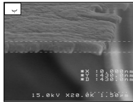
شکل ۲. تصاویر FESEM از نانولوله‌های اکسید تیتانیوم سنتز شده به روش اکسیداسیون آندی در الکترولیت آبی حاوی ۱٪ وزنی اسید
