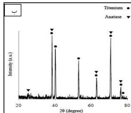
شکل ۱. الگوهای XRD مربوط به نانولوله‌های سنتز شده در (الف) الکترولیت آلی و (ب) الکترولیت آبی که به مدت ۳ ساعت در دمای ۴۸۰°C آنیل شدند.
