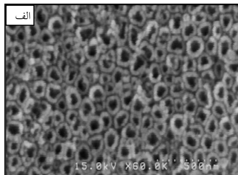
شکل ۲. تصاویر FESEM از نانولوله‌های اکسید تیتانیوم سنتز شده به روش اکسیداسیون آندی در الکترولیت آبی حاوی ۱٪ وزنی اسید
