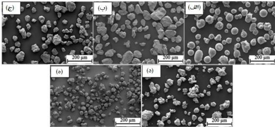
شکل ۱. تصویر میکروسکوپی الکترونی روبشی از الف) پودر تجاری، ب) ۰ % YSZ، ج) ۵ % YSZ، د) ۱۰ % YSZ، ه) ۱۵ % YSZ
