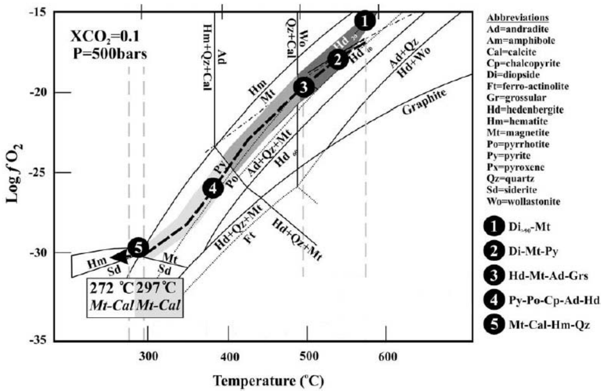
شکل ۴. نمودار T-LogfO 2 (تغییر یافته بعد از [۱۶] که محدوده پایداری کانیه‌های کالک‌سیلیکاته اسکارنی، اکسیدها، سولفیدها و کانیه‌های کربناته را نشان می‌دهد [۱۹].
