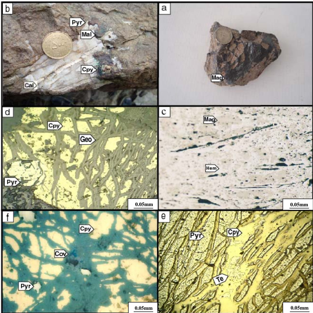
شکل ۳. تصاویر ماکروسکوپی، صحرایی و میکروسکوپی (در نور Xp ) از کانی‌سازی اسکارن کم‌تال. (a) تصویر نمونه دستی کانی‌سازی رگه‌ای مگنتیت در زون برشی شده. (b) تصویر صحرایی از پیریت یوهدرال همراه با کلسیت بلورین و کالکوپیریت. (c) مارتیتی شدن مگنتیت در اثر فرآیندهای سوپرژن در محیط اکسیدان. (d) جانشینی پیریت توسط کالکوپیریت، و دگرسانی کالکوپیریت به گوتیت از محل شکستگی‌ها. (e) کانی تتراهدريت در داخل کالکوپیریت. (f) کانی کوولیت در داخل شکستگی‌های کالکوپیریت. (Mag = مگنتیت؛ Hem = هماتیت؛ Geo = گوتیت؛ Pyr = پیریت؛ Cpy = کالکوپیریت؛ Cov = کوولیت؛ Te = تتراهدريت؛ Mal = ملاکیت؛ Az = آزوریت).
