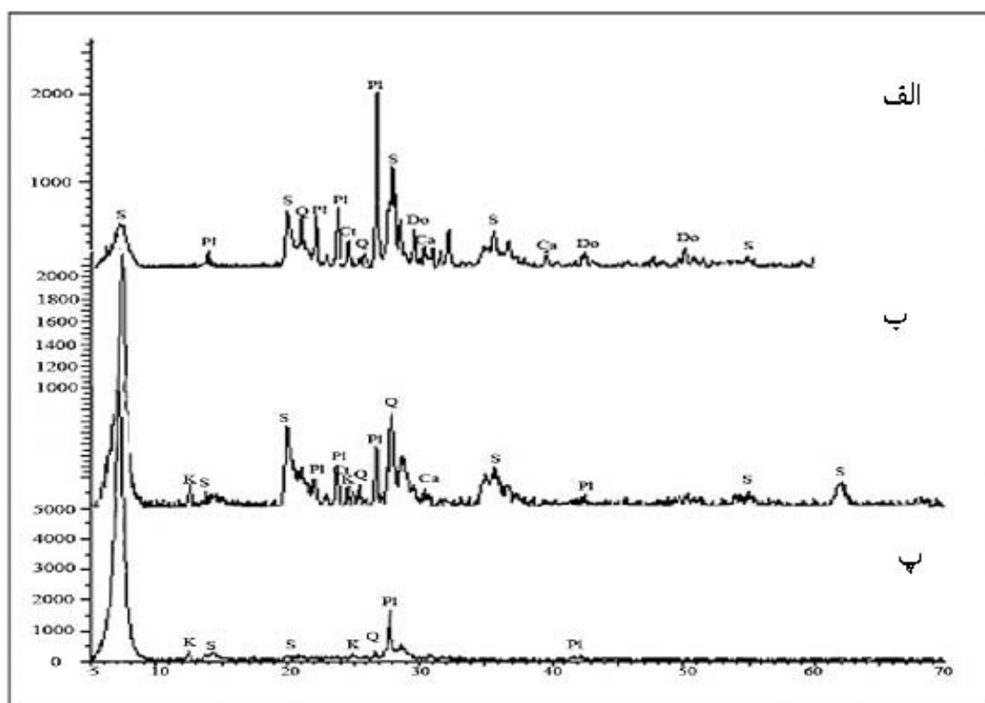
شکل ۴. نتایج آنالیز XRD در نمونه‌های رسی برداشت شده از نمونه خام معدنی (الف)، ذرات کوچکتر از ۲ میکرون (ب)، و مقطع جهت دار (پ) =S اسمکتیت، Q= کوارتز، K= کائولینیت، PI= پلاژیوکلاز، Ca کلسیت، CT= اپال و Do= دولومیت.
