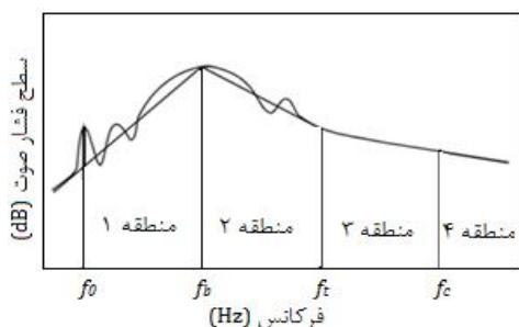
شکل ۲ محدوده فرکانسی نویز پروانه در حالت کابیناسیونی [۴]
