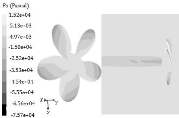
شکل ۷- الف کانتور فشار استاتیک جهت محاسبه عدد کایتاسیون در J=0.12
