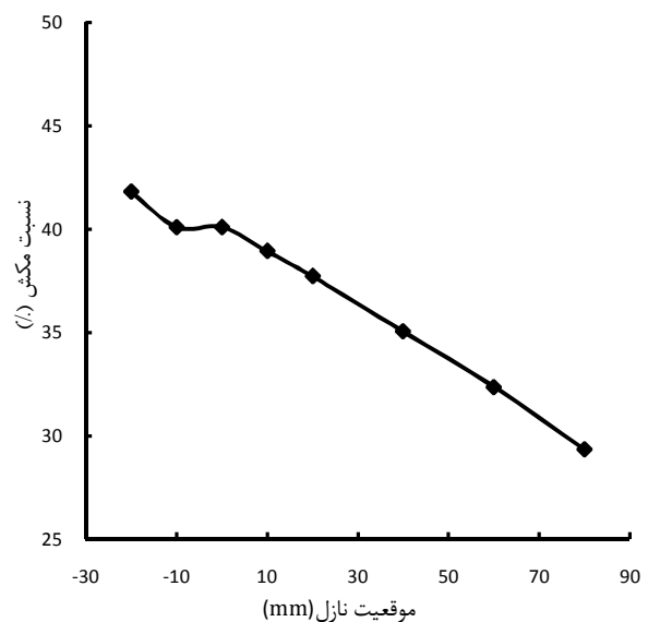
شکل ۴ تغییر نسبت مکش بحرانی با موقعیت نازل در دمایی مولد 115^{\circ}\text{C} و دمایی اواپراتور 5^{\circ}\text{C}
