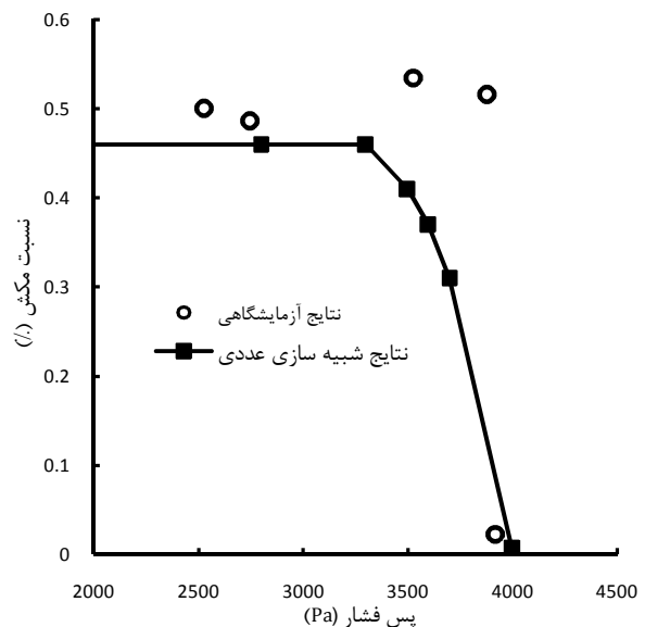
شکل ۳ تغییر نسبت مکش در پس فشارهای مختلف در دمایی اواپراتور 7/5^{\circ}\text{C}
