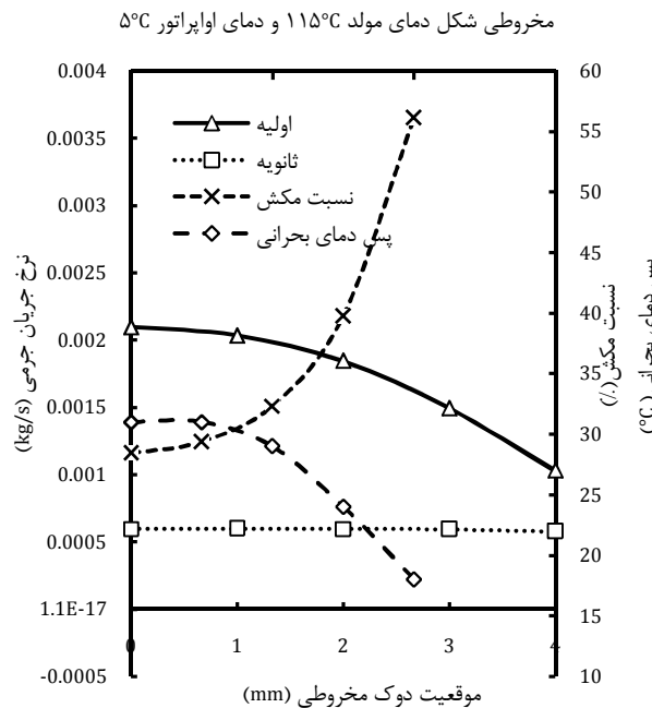
شکل ۱۳ تغییر دبی جرمی اولیه، ثانویه نسبت مکش و دمای بحرانی با موقعیت دوک مخروطی شکل دمای مولد ۱۱۵°C و دمای اوپراتور ۵°C
