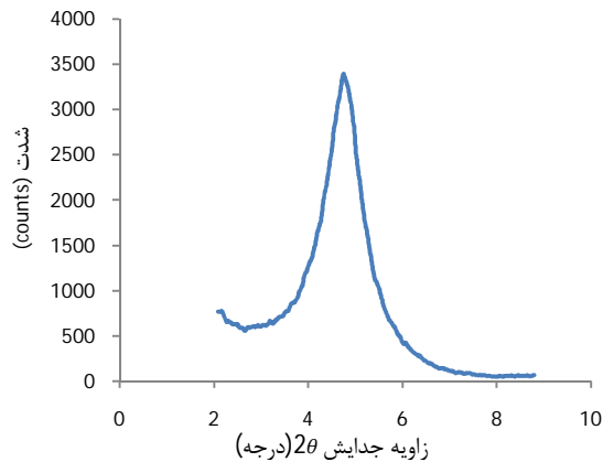
الف) منحنی پراش اشعه ایکس کلوئیدیسی
