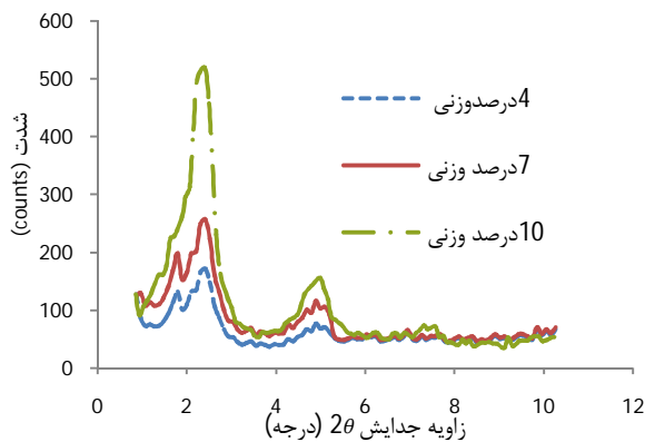
ب) منحنی پراش اشعه ایکس رزین اپوکسی
