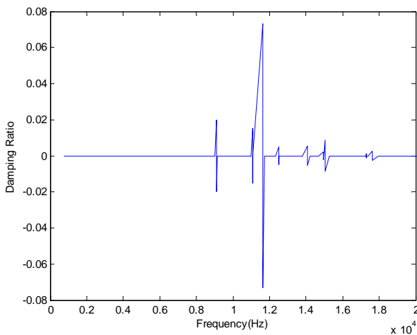
شکل ۶- نمودار ضریب استهلاک برای سیستم ترمز سمند
