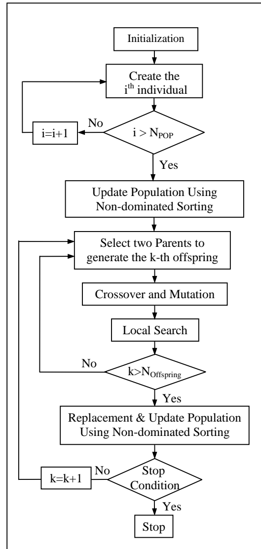
شکل ۱۰- الگوریتم MARCOMA
