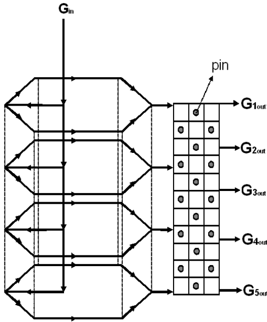
شکل ۸- گراف پره در حالت سه بعدی
