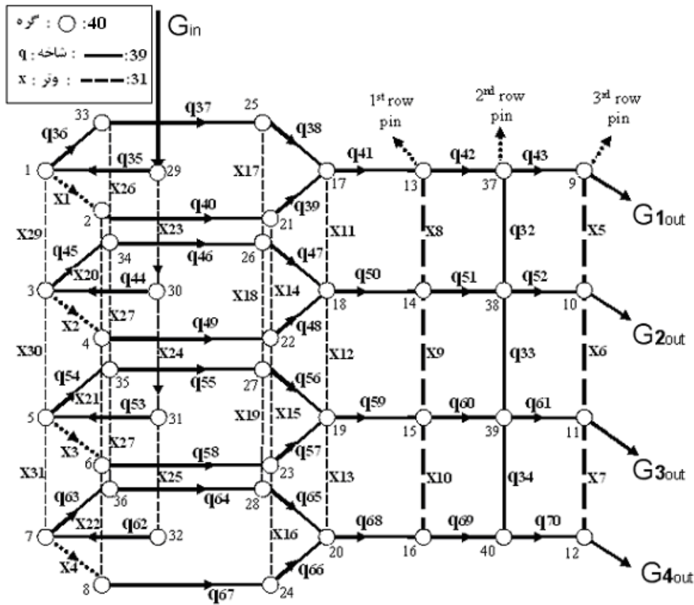
شکل ۱۰- گراف پره مورد مطالعه
