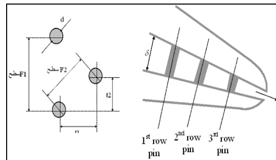
شکل ۹- چیدمان پین‌ها در لبه خروجی
