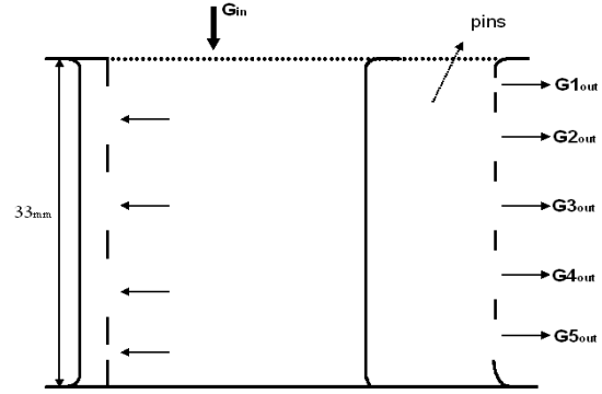
شکل ۵- مقطع عمودی پره
