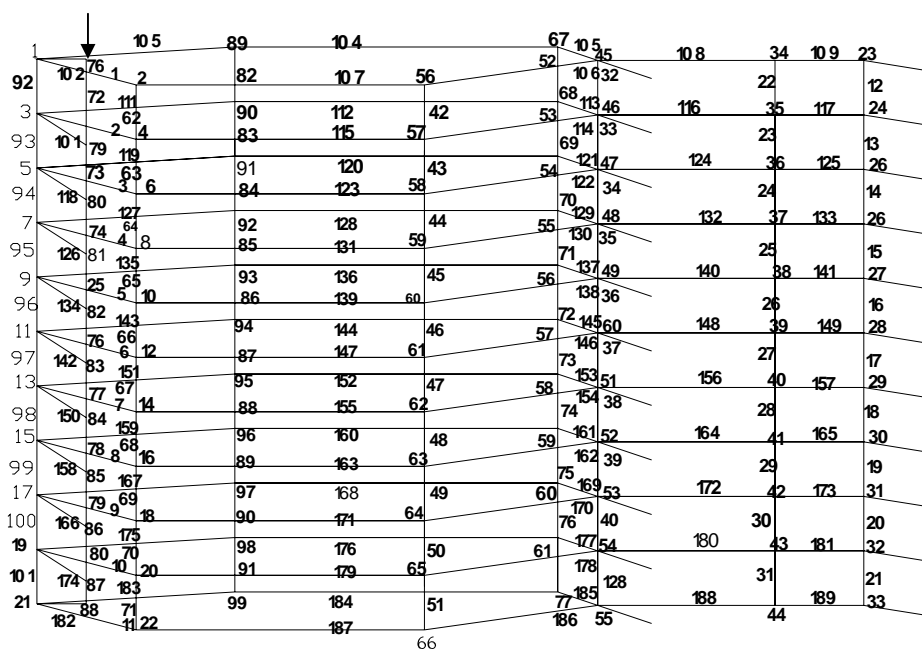
شکل ۱۴- شبکه‌بندی هیدرولیکی پره استاتور
