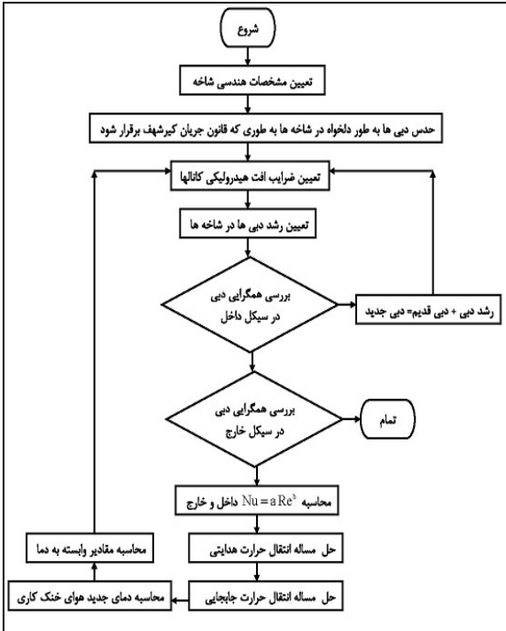
شکل ۳- الگوریتم محاسبات ترموهیدرولیک
