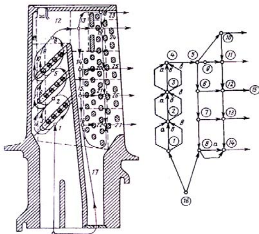
شکل ۲- شبکه هیدرولیکی کانال‌های خنک‌کاری یک پره [۷]
