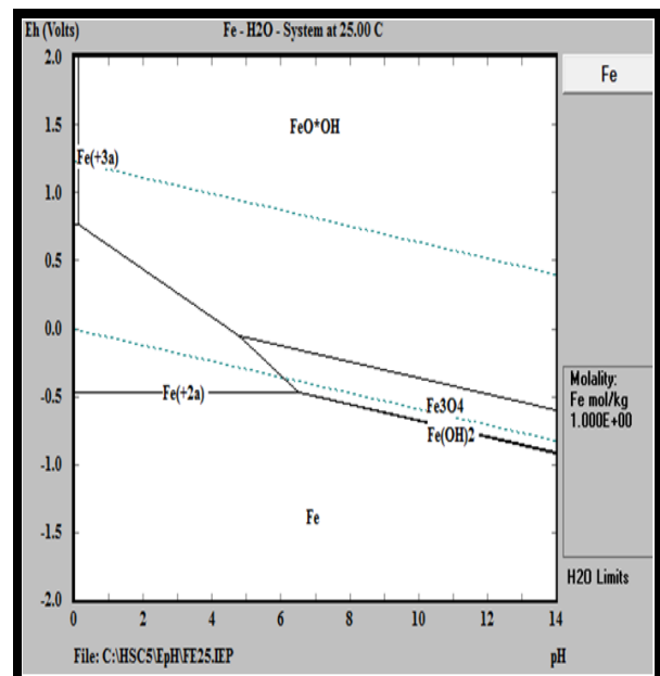
شکل (۱): نمودار پوربه آهن (ترسیم شده توسط نرم افزار HCS)
