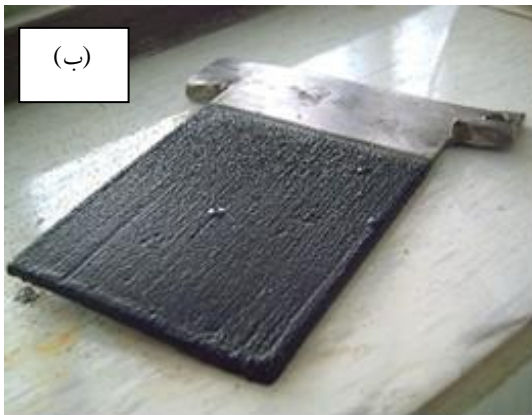
شکل (۲): (الف): رسوب تولید شده در pH ۳، (ب): رسوب تولید شده در
