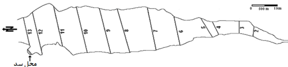
شکل ۱- نمای بالایی آبنگير سد پانزده‌ی خرداد و محل قرارگیری مقاطع عرضی.
