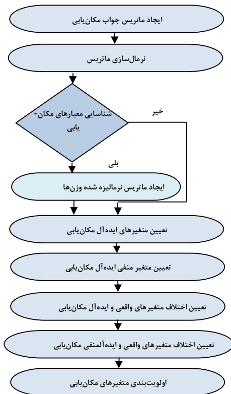
شکل ۴. مراحل اجرای روش TOPSIS در قالب مکان یابی
