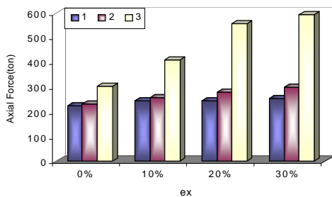
شکل ۲: نیروی محوری فشاری ستون شماره ۱ در سازه دارای جداگر تیپ ۱ تحت زلزله بم.
