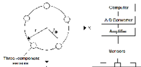
شکل ۶: نحوه اندازه‌گیری میکروترومورها در روش آرایه‌ای.
