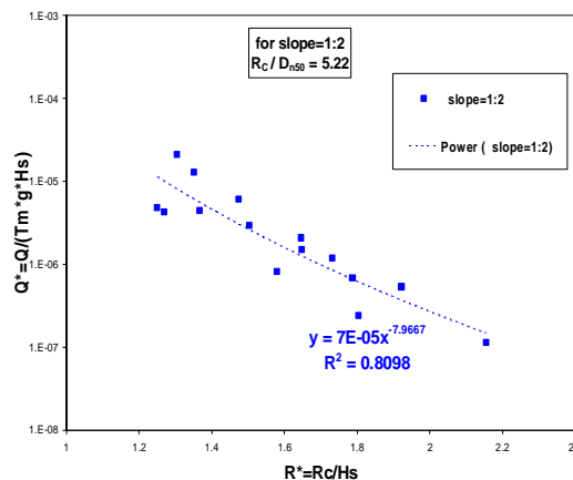
شکل ۱۰: نمودار همبستگی داده‌ها در شیب ۱:۲
