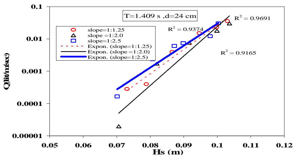
شکل ۸: نمودار Q بر حسب H_s ، به تفکیک شیب سازه، برای عمق آب ۲۴ سانتیمتر و پریرود حداکثر ۱/۴۰۹ ثانیه.
