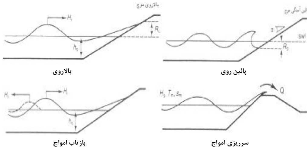
شکل ۱: واکنش‌های هیدرولیکی سازه‌های ساحلی.
