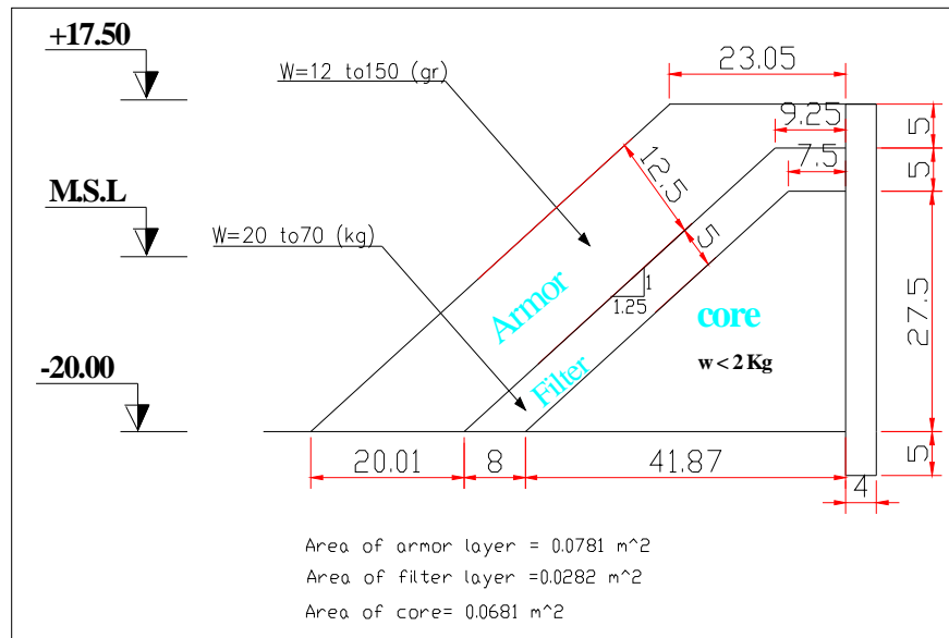
شکل ۳: مقطع عرضی مدل دیوار ساحلی با شیب ۱:۲۵. ۱.
