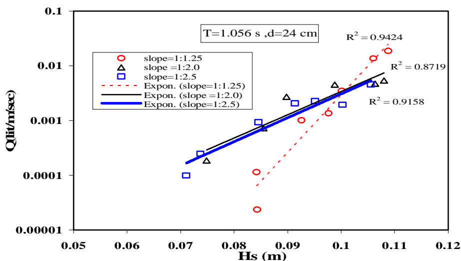
شکل ۷: نمودار Q بر حسب H_s ، به تفکیک شیب سازه، برای عمق آب ۲۴ سانتیمتر و پریرود حداکثر ۱/۰۵۶ ثانیه.
