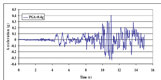
شکل ۱۲: شتاب‌نگاشت افقی زلزله‌ی طبس فیلتر شده برای فرکانس ۱۵ هرتز و کالیبره شده برای 0.4g .
