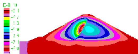
شکل ۴-الف: کنتورهای نشست در پایان ساخت - سد با هسته مایل.
