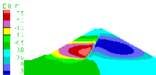
شکل ۵-الف: کنتورهای تغییر مکان افقی در پایان ساخت - سد با هسته مایل.
