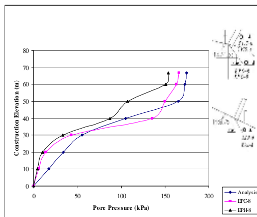
شکل ۹: تغییرات فشار آب حفره ای در کف هسته در طول زمان ساخت سد-مقایسه بین مقادیر محاسباتی و مقادیر ابزار دقیق.
