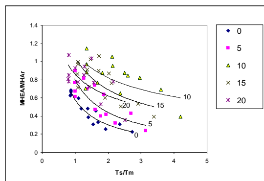
شکل 12: نمودار حداکثر شتاب نرمال شده به پیوند نوسانی نرمال شده برای زوایای مختلف سنگ بستر با افق.
