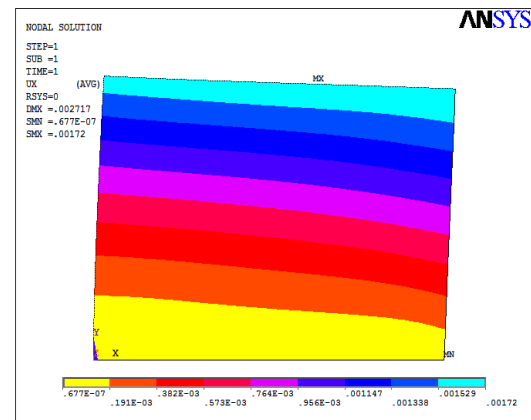
شکل 9: توزیع تغییر شکل افقی در دو حالت دقیق و همگن شده.
