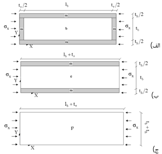
شکل 7: مراحل مربوط به فرآیند همگن‌سازی.
