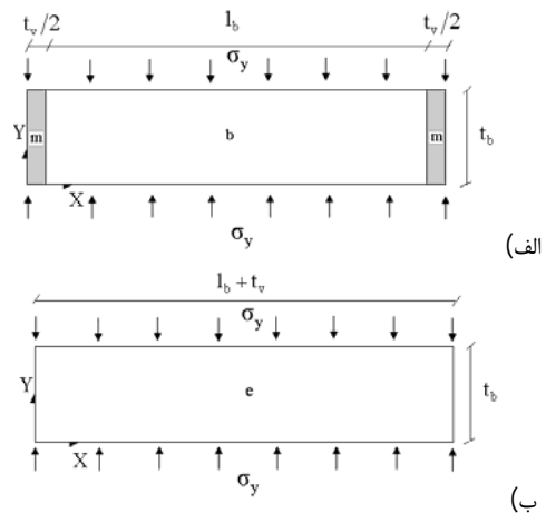
شکل 8: مراحل مربوط به فرآیند همگن‌سازی.
