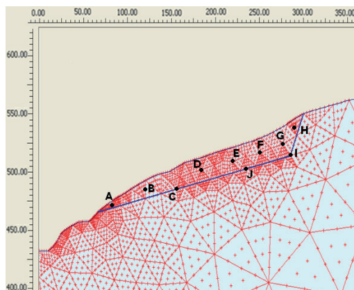
شکل (۱۰): بخشی از مدل مش بندی شده در شکل (۹) به همراه جانمایی نقاط گزینش شده برای دریافت پاسخ لرزه‌ای
