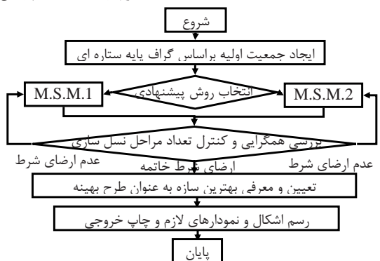
شکل ۴ کلیات بهینه بایی مقاطع و توپولوژی خرپاها بر اساس روش های جستجوی چند منظوره
