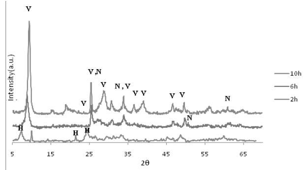
شکل ۱- طیف XRD نمونه‌های حاوی ۰/۵ گرم EDTA در سه زمان مختلف.
