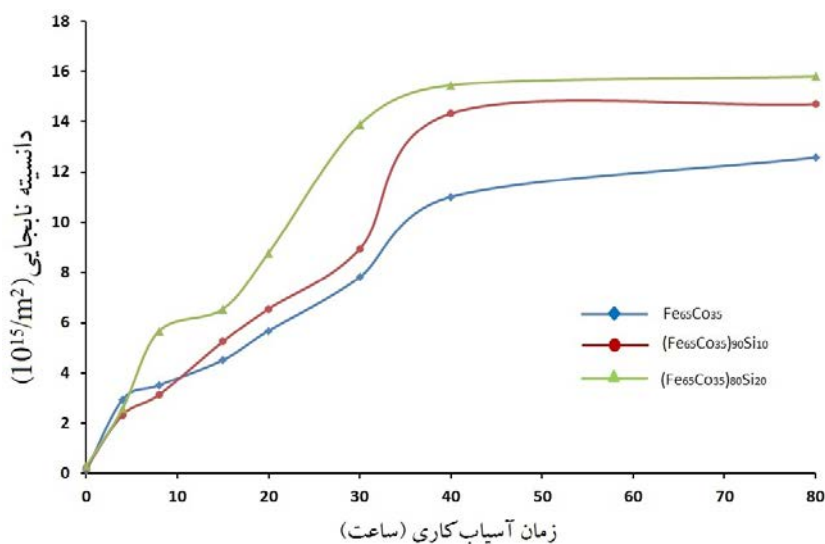
شکل ۷- منحنی تغییرات دانشیه نابجایی برای سه ترکیب حاوی ۰، ۱۰ و ۲۰٪ سیلیسیم در زمان‌های مختلف آسیاب کاری
