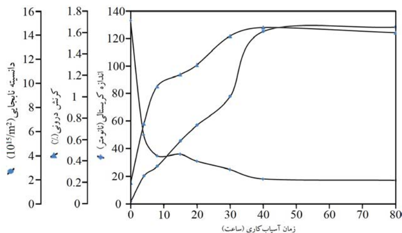
شکل ۸- تغییرات دانسیته‌ی نابه‌جایی، اندازه‌ی دانه و میکرو کرنش شبکه در زمان‌های مختلف آسیاب‌کاری
