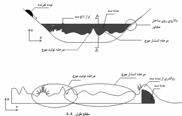
شکل (۱): مراحل تولید، انتشار، بالاروی و روگذری امواج ضربه ای ناشی از زمین لغزش در مخازن سد [۳]
