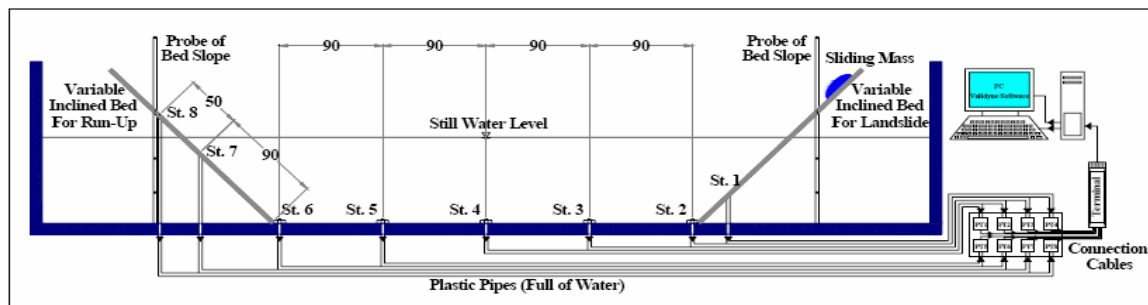
شکل (۳): شمایی از تنظیمات کلی آزمایشات شامل اجزای آزمایش، سیستمهای اندازه گیری، ارتباط بخشهای مختلف و موقعیت دقیق استقرار حساسه ها (کلیه ابعاد به سانتی متر است) [۷]
