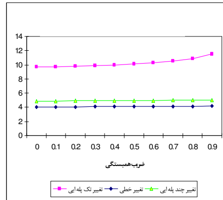
شکل ۴. متوسط طول دنباله شبکه ۱ برای انواع تغییرات
