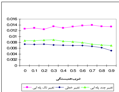
شکل ۵. نرخ خطا در شبکه ۳ برای انواع تغییرات
