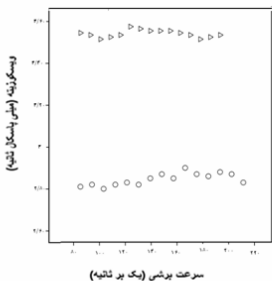
شکل ۱ نسبت ویسکوزیته به سرعت برشی در عصاره‌های استخراجی (a) و نسبت تنش به سرعت برشی در عصاره‌های استخراجی b توسط اتوکلاو ۲۰ درجه سانتی گراد و اتوکلاو ۱۰۰ درجه سانتی گراد
