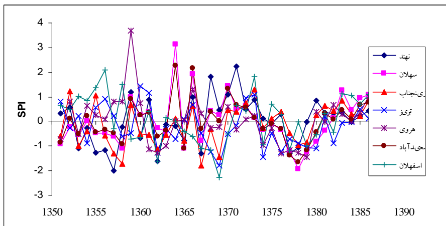
شکل ۳: نمودار تغییرات شاخص SPI در دشت تبریز (۱۳۵۱-۸۶) مأخذ: نگارندگان
