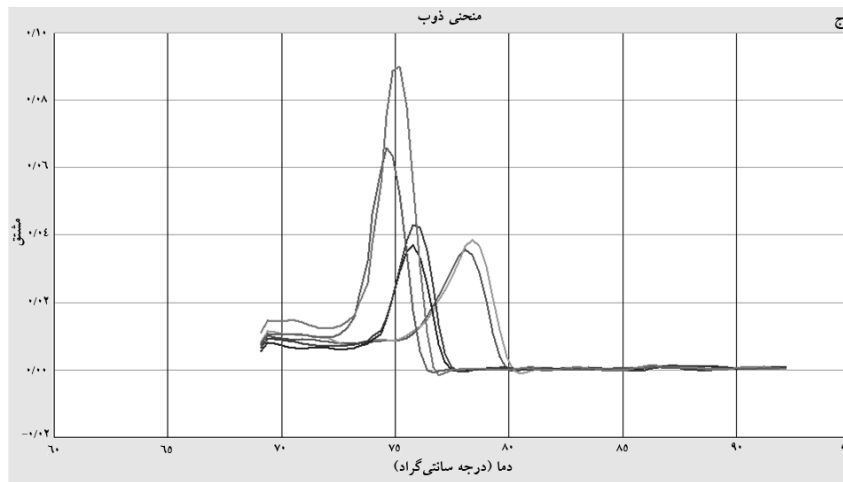
شکل ۴ الف) آنالیز منحنی ذوب برای ژن‌های DSCAM، DYRK1A2 و PMP22 در نمونه‌های تخلیص شده با کیت (Qiagen) QIAamp DNA Micro، ب) آنالیز منحنی ذوب برای ژن‌های DSCAM، DYRK1A2 و PMP22 در نمونه‌های تخلیص شده با روش جوشاندن، ج) آنالیز منحنی ذوب برای ژن‌های DSCAM، DYRK1A2 و PMP22 در نمونه‌های تخلیص شده با کیت DNP™ (سینازن)
