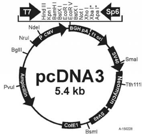
شکل ۱ نقشه ژنتیکی پلاسمید یوکاریوت بیانی pcDNA3
