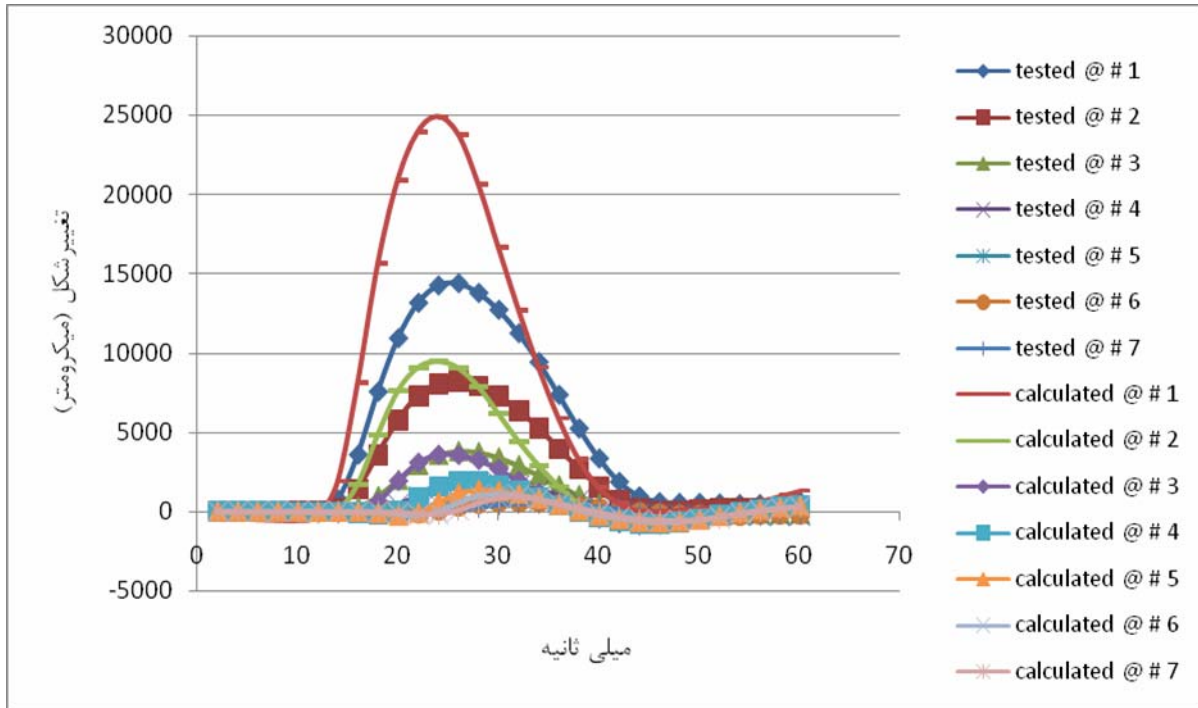
شکل ۶. تاریخچه‌های زمانی تغییرشکلی اندازه گیری و محاسبه شده- RMSE بالا و خطای پیک قابل ملاحظه است.
