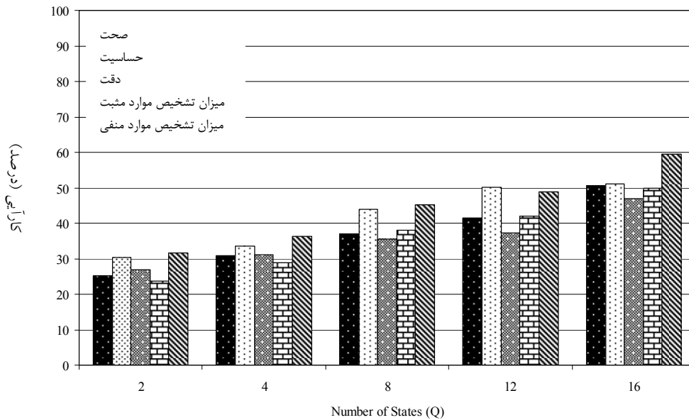
شکل ۴- ارزیابی عملکرد الگوریتم ترکیبی HMM-MLP تعداد وضعیت‌های پنهان ۵ سیگنال‌های عاری از مؤلفه P300 با ۵ مرتبه متوسط‌گیری از سیگنال‌ها و انتخاب ۳ عدد تابع گوسین برای تخمین تابع توزیع احتمال مشاهدات مدل.
