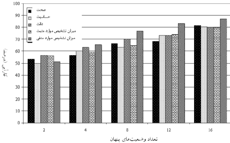
شکل ۲- ارزیابی عملکرد الگوریتم ترکیبی HMM-MLP در تفکیک سیگنال‌های حاوی مؤلفه P300 از سیگنال‌های عاری از مؤلفه P300 با ۱۵ مرتبه متوسط‌گیری از سیگنال‌ها و انتخاب ۳ عدد تابع گوسین برای تخمین تابع توزیع احتمال مشاهدات مدل.
