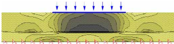
شکل ۷- ماکزیمم تنش برشی برای وزن 400 گرم اعمالی به صورت یکنواخت بر دیسک
