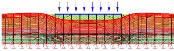
شکل ۶- جابجایی در زیر دیسک با بزرگنمایی \times 20
