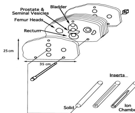
شکل ۳- طرح کلی فانتوم ناهمگن لگن ساخته شده
