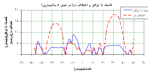
شکل ۶ - اختلاف دوز و DTA حاصل از پروفایل ها
