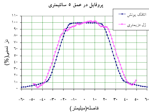
شکل ۵ - پروفایل های به دست آمده از دوزیمتر اتاقک یونش و ژل دوزیمتری در عمق ۵ سانتیمتری
