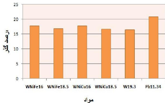
شکل ۹- درصد گذر برای ضخامت ۶/۵ سانتیمتر از مواد مختلف
