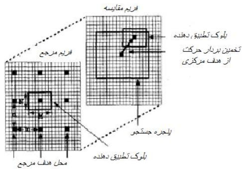
شکل ۱- نمایشی از تطبیق بلوکی
