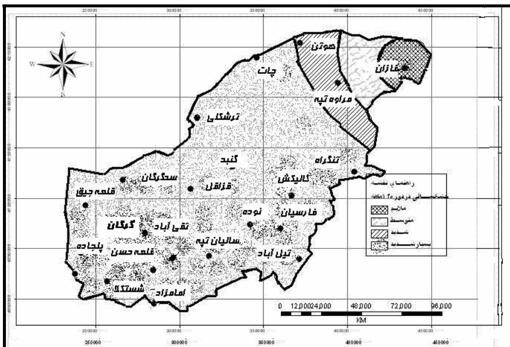
شکل ۶- نقشه‌ی وضعیت خشکسالی در مقیاس زمانی ۱۲ ماهه در استان گلستان
