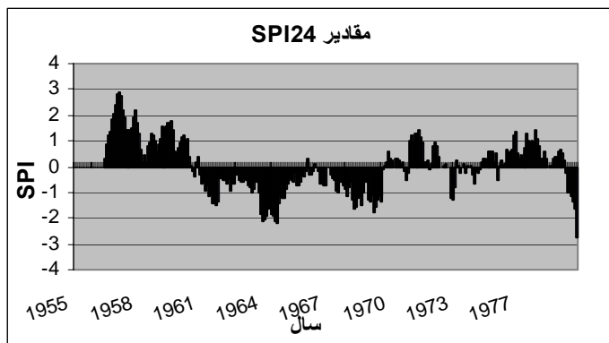
شکل ۳- نمودار خشکسالیها و ترسالیهای ایستگاه تقی آباد (نمونه) در مقیاس های زمانی مورد مطالعه (۶، ۹، ۱۲ و ۲۴ ماهه)
