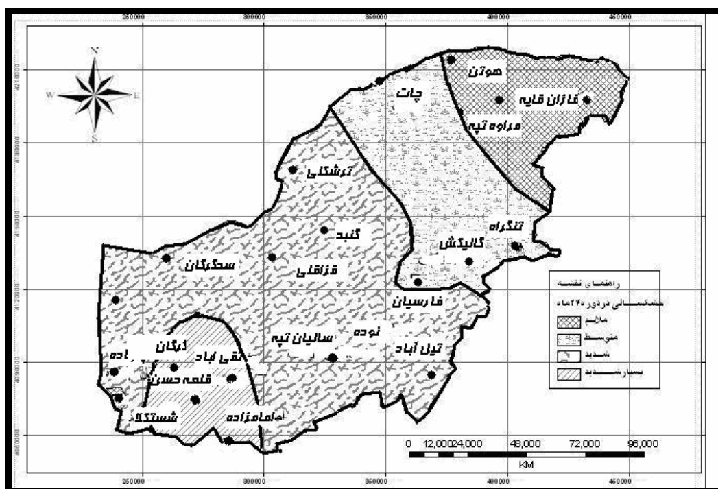
شکل ۷- نقشه‌ی وضعیت خشکسالی در مقیاس زمانی ۲۴ ماهه در استان گلستان
