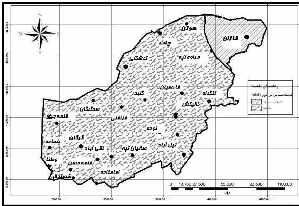
شکل ۴- نقشه ی وضعیت خشکسالی در مقیاس زمانی ۶ ماهه در استان گلستان
