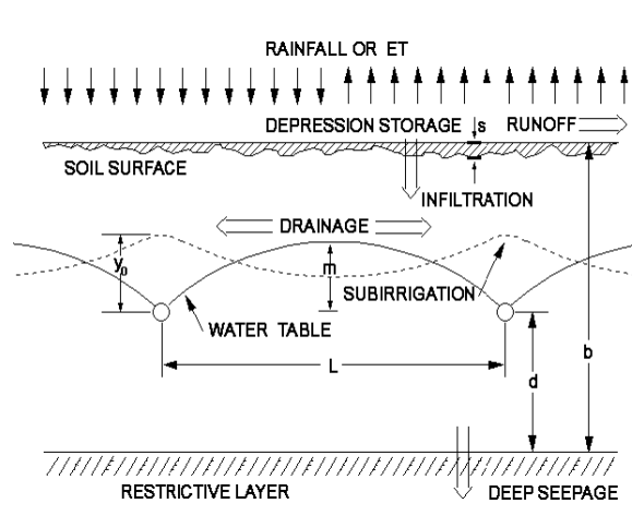
شکل 1- شرح تصویری مدل در رابطه با پارامترهای بیلان آبی
